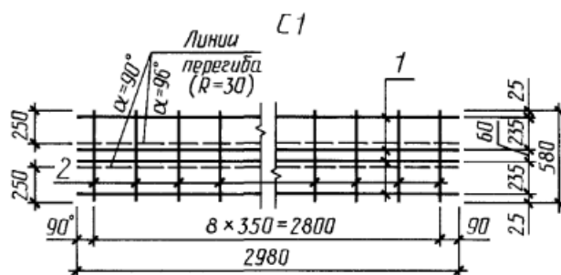
Арматурные сетки С1 и С2
