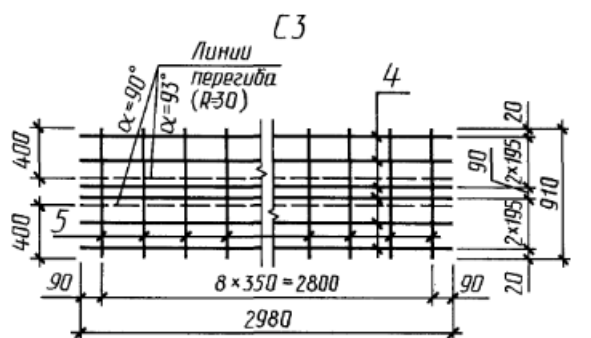
Арматурные сетки С3 и С4
